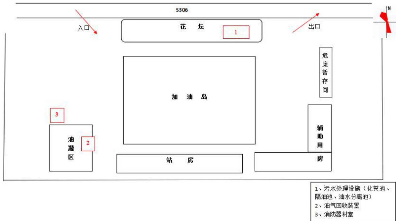
附图2 建设项目厂区平面布局图
