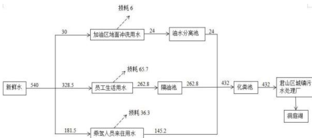
图 3.5-1 项目水平衡图 (单位 m^3/d )
