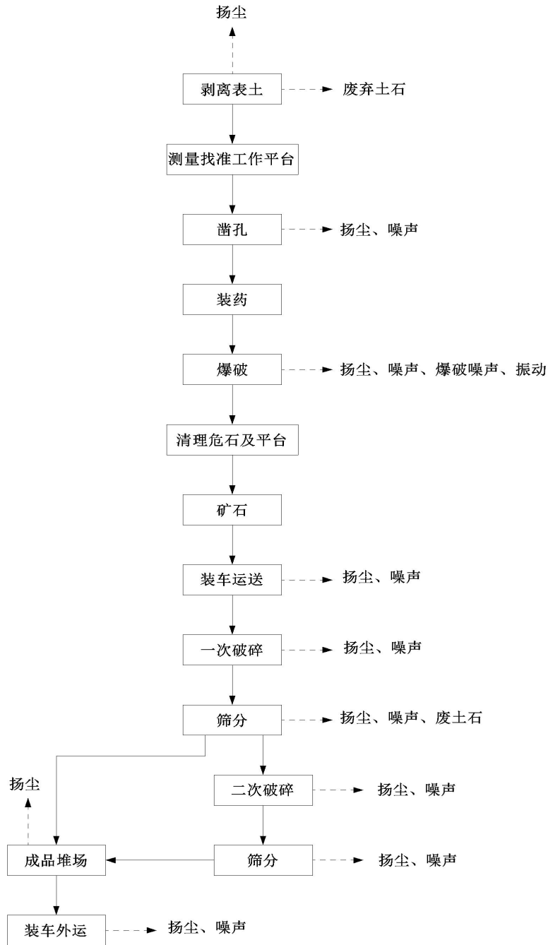
图 4.1-1 项目矿石开采、加工过程工艺流程及产污节点图
