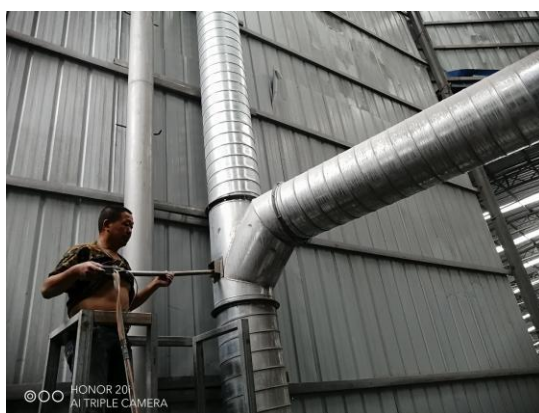
(破碎) 有组织废气出口
