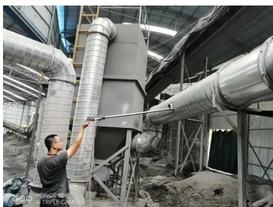
(破碎) 有组织废气进口
