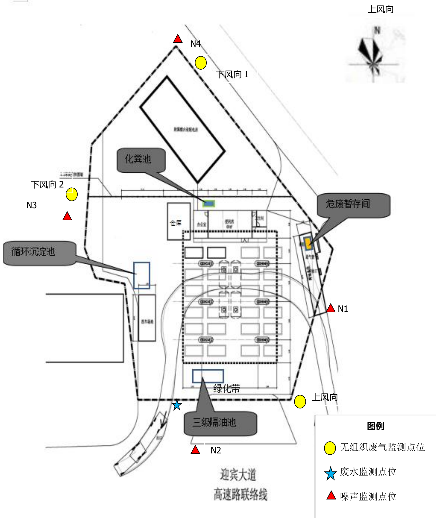
附图 2 项目平面布局及监测布点图
