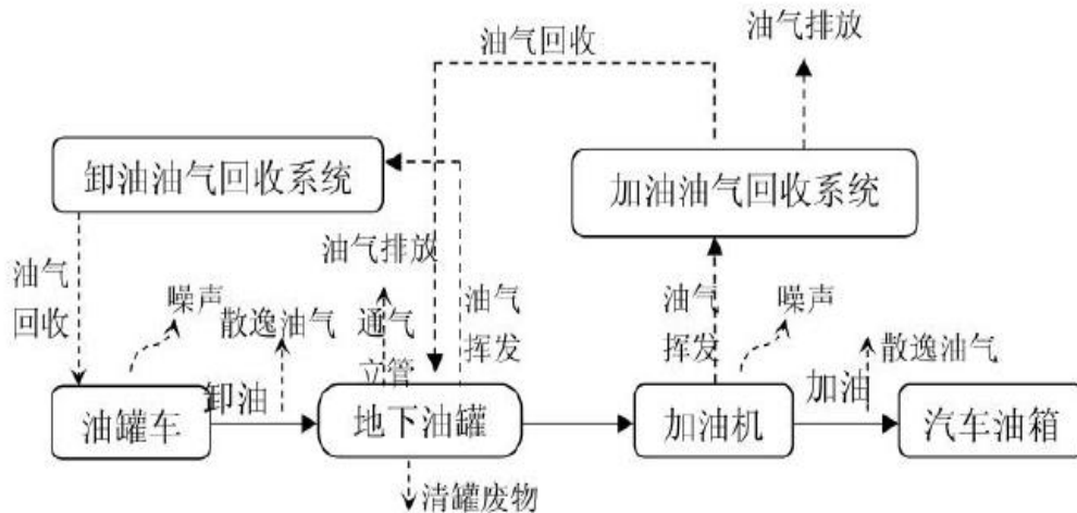
图 5-1 加油工艺流程及产污环节图
