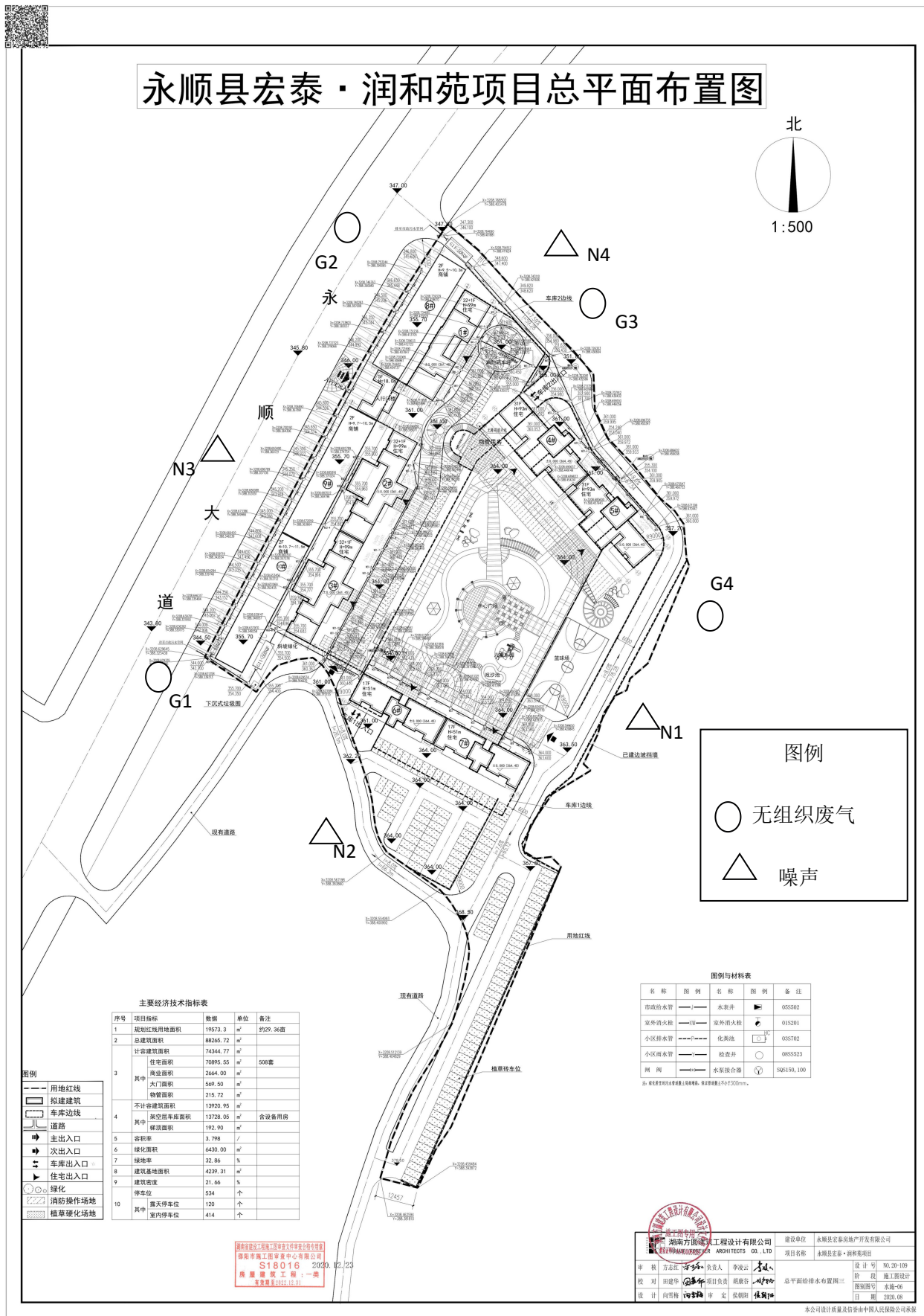
附图2 项目总平面图及监测点位图
