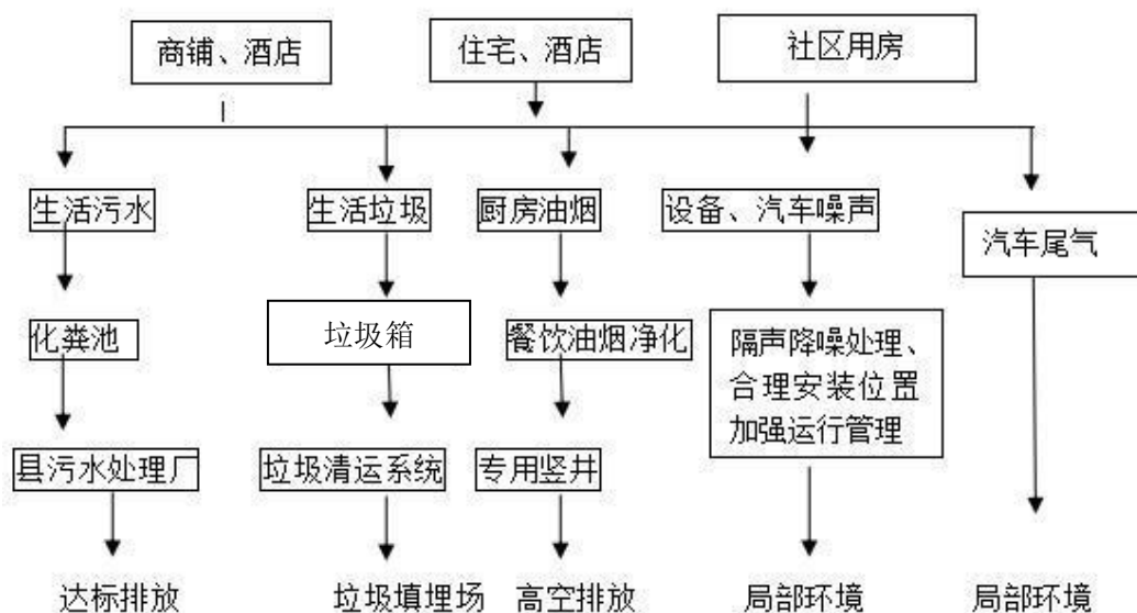
图 3-1 营运期基本工序及污染工艺流程图
