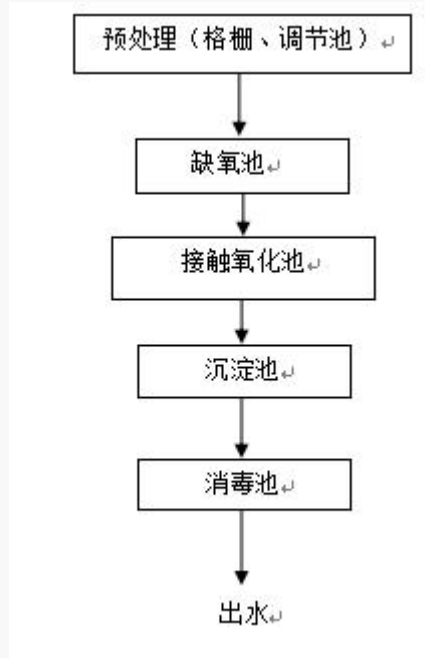
图3-3 污水处理工艺图
